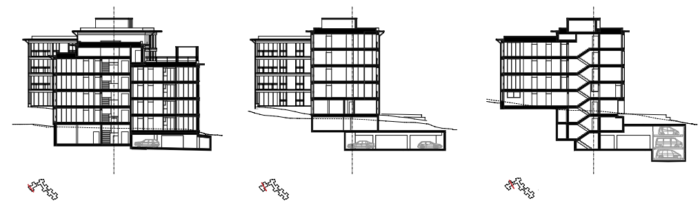
Querschnitte Haus Rötelstrasse
