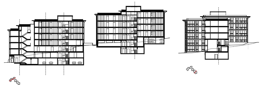
Schnitt Rötelstrasse - Seminarstrasse 103
