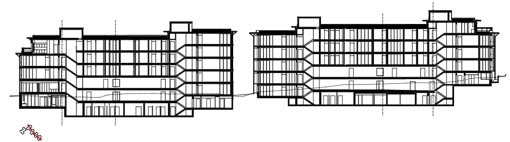
Längsschnitt Seminarstrasse 97-103
