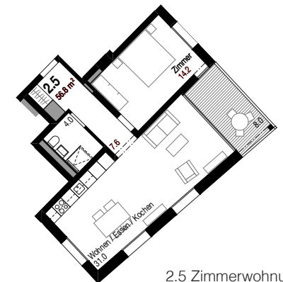
2.5 Zimmerwohnung Seminarstrasse 97
